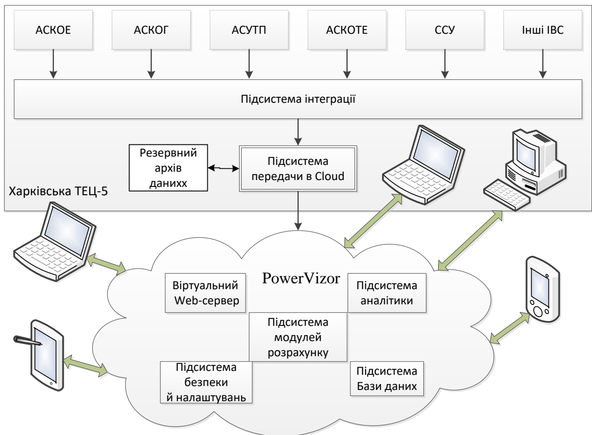
Рисунок 1 - Логічна архітектура PowerVizor
